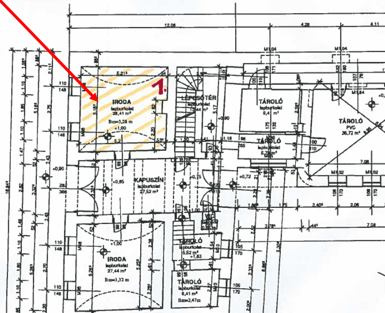
FÖLDSZINT FELMÉRÉSI ALAPRAJZA M 1:100
