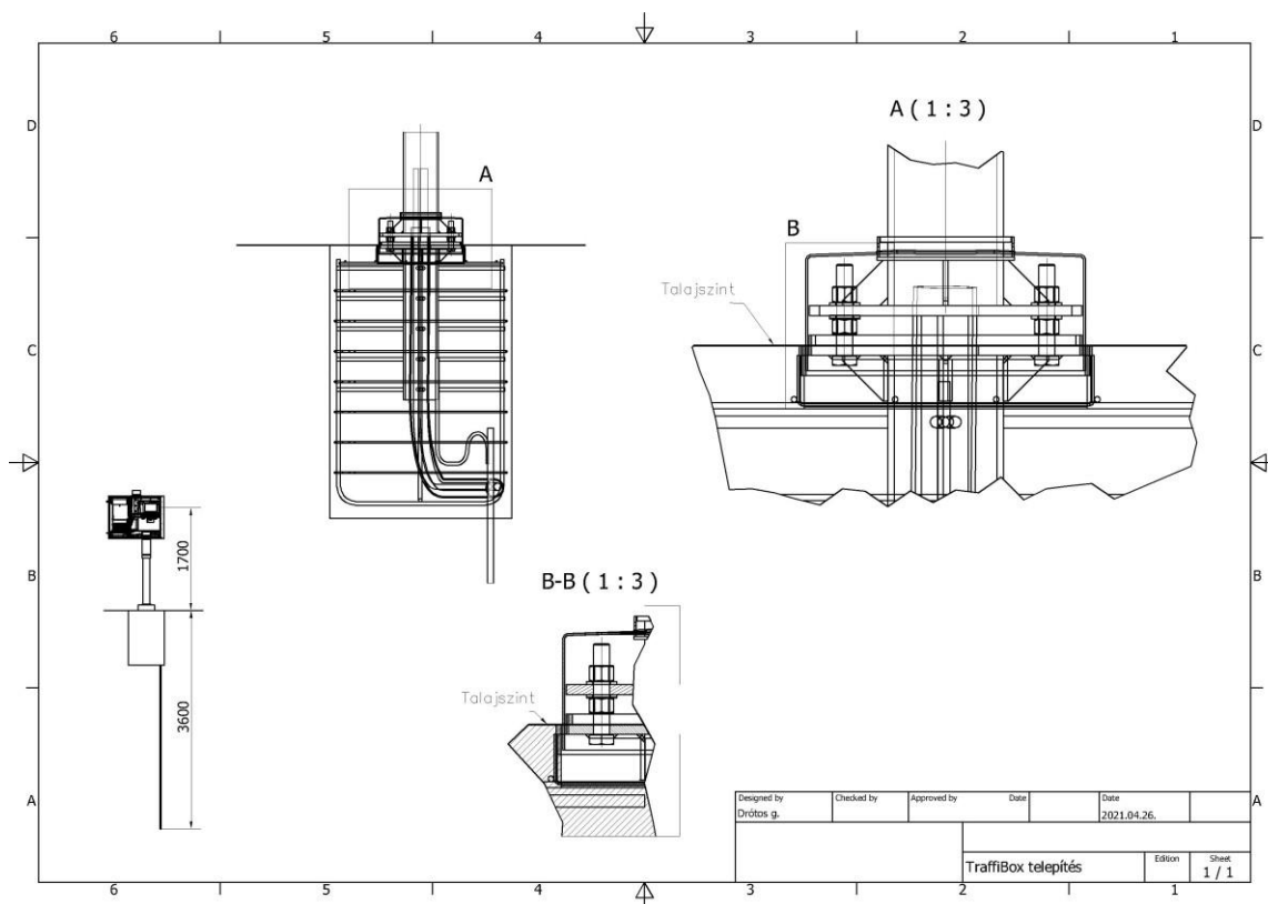
3. Szekrény telepítési elrendezése
