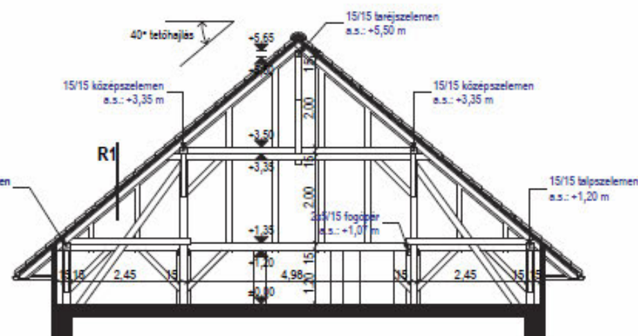
B-B metszet
