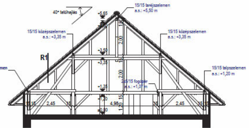
B-B metszet
