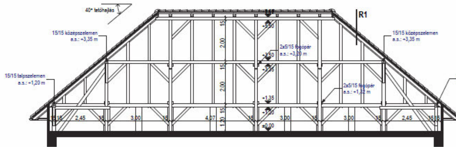
A-A metszet
